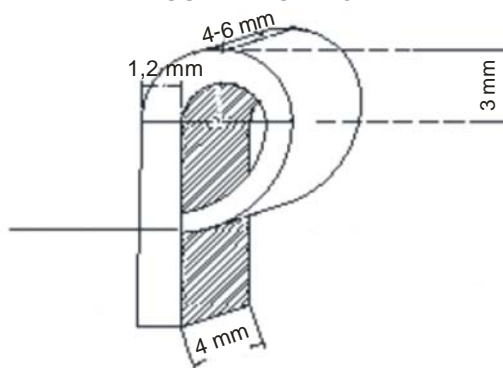
Sl. 12 Dimenzije i savitljivost sablje
