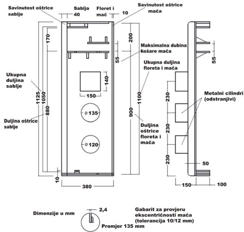
Gabariti za kontrolu oružja
